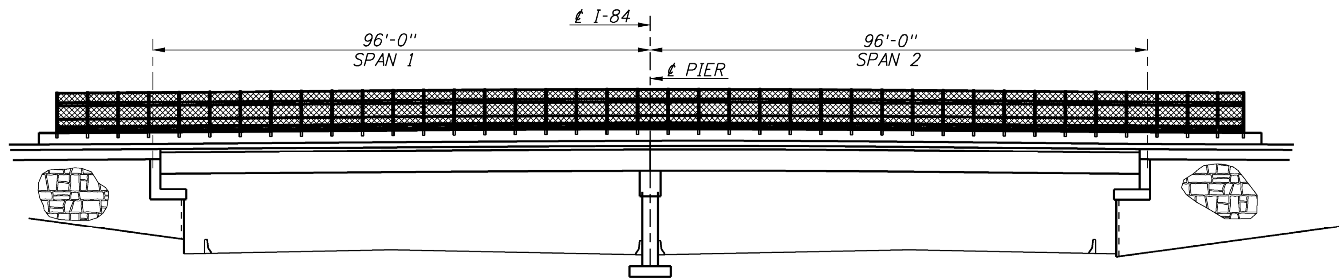
ELEVATION
